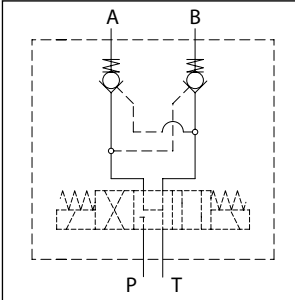
BLOCCO 08 (Manifold 08)
