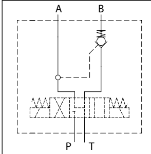
BLOCCO 07 (Manifold 07)
