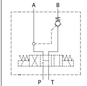
BLOCCO 27 (Manifold 27)
