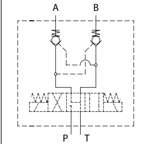
BLOCCO 26 (Manifold 26)
